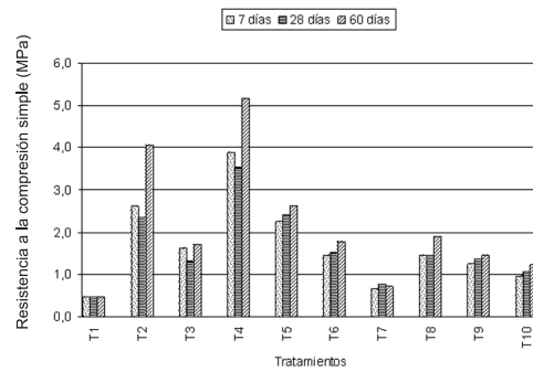
Figura 3. Valores de la resistencia a la compresión simple de los ladrillos confeccionados a partir de mezclas de suelo-cemento-cáscara
